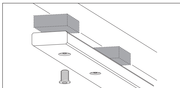
Illustration détaillée de la façon de placer les pièces de remplissage entre la poutre de bois et le plafond.
